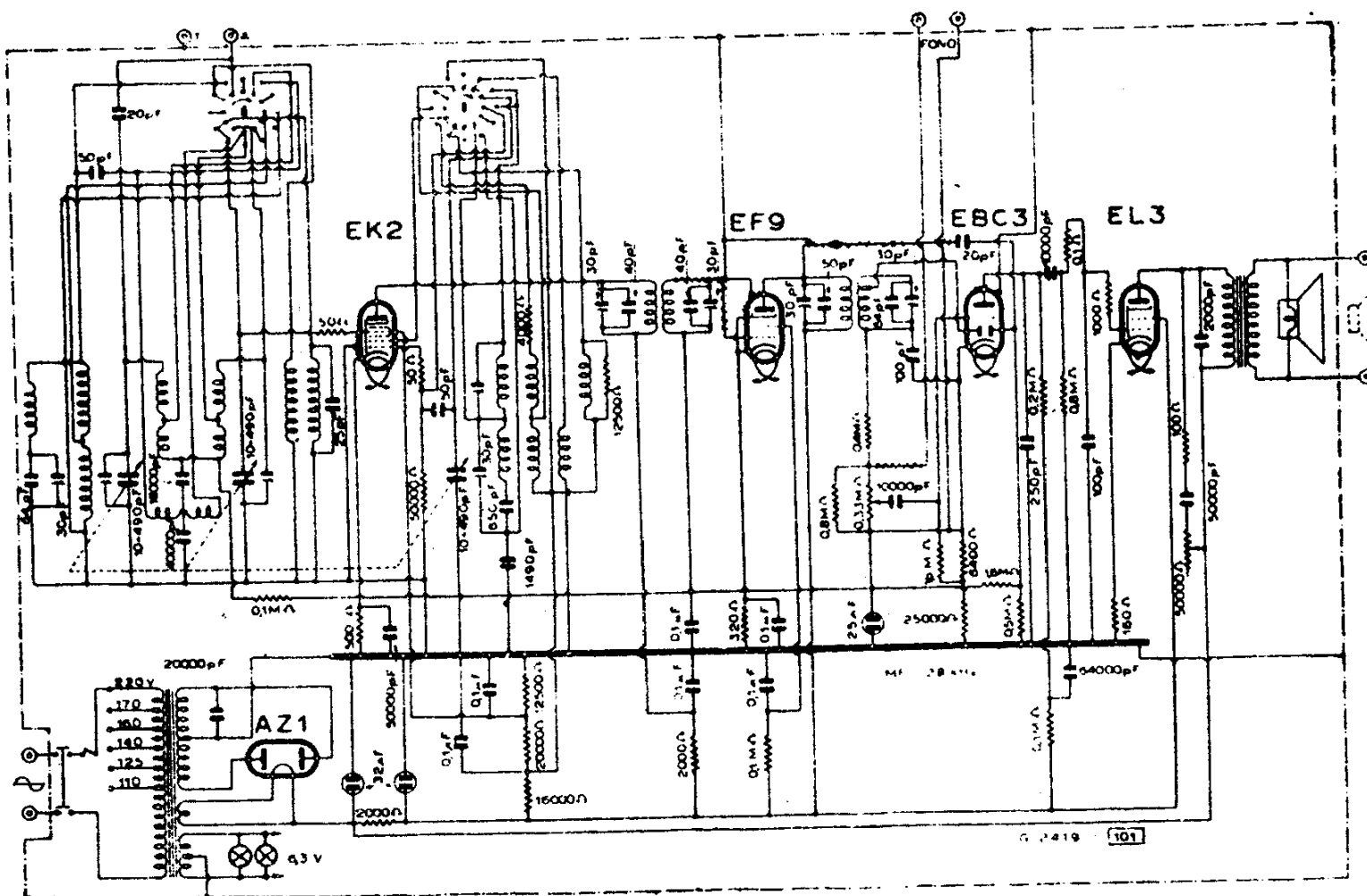
PHILIPS RADIO - MODD. « 461 E » « 469 E - FONO »
